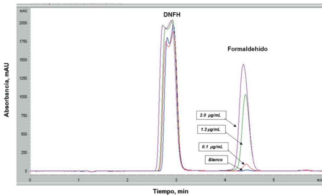
Figura 2. Cromatogramas obtenidos por CLAR para el blanco y diferentes concentraciones del estándar de formaldehído: 0,1 µg/mL, 1,2 µg/mL y 2,0 µg/mL
