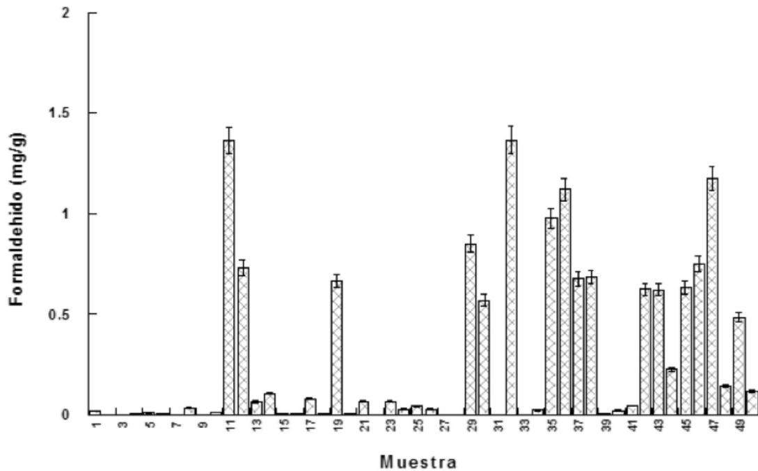
Figura 4. Contenido de formaldehído libre (mg/g) determinado en cincuenta muestras comerciales de esmaltes de uñas
