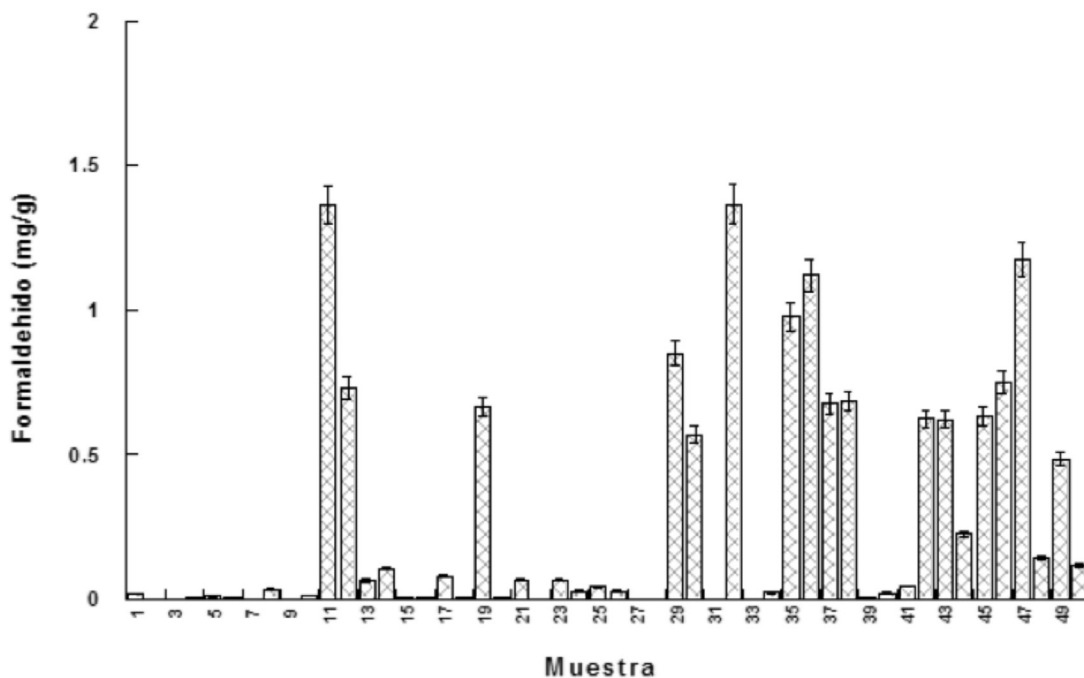
Figura 4. Contenido de formaldehído libre (mg/g) determinado en cincuenta muestras comerciales de esmaltes de uñas Fuente: elaboración propia
