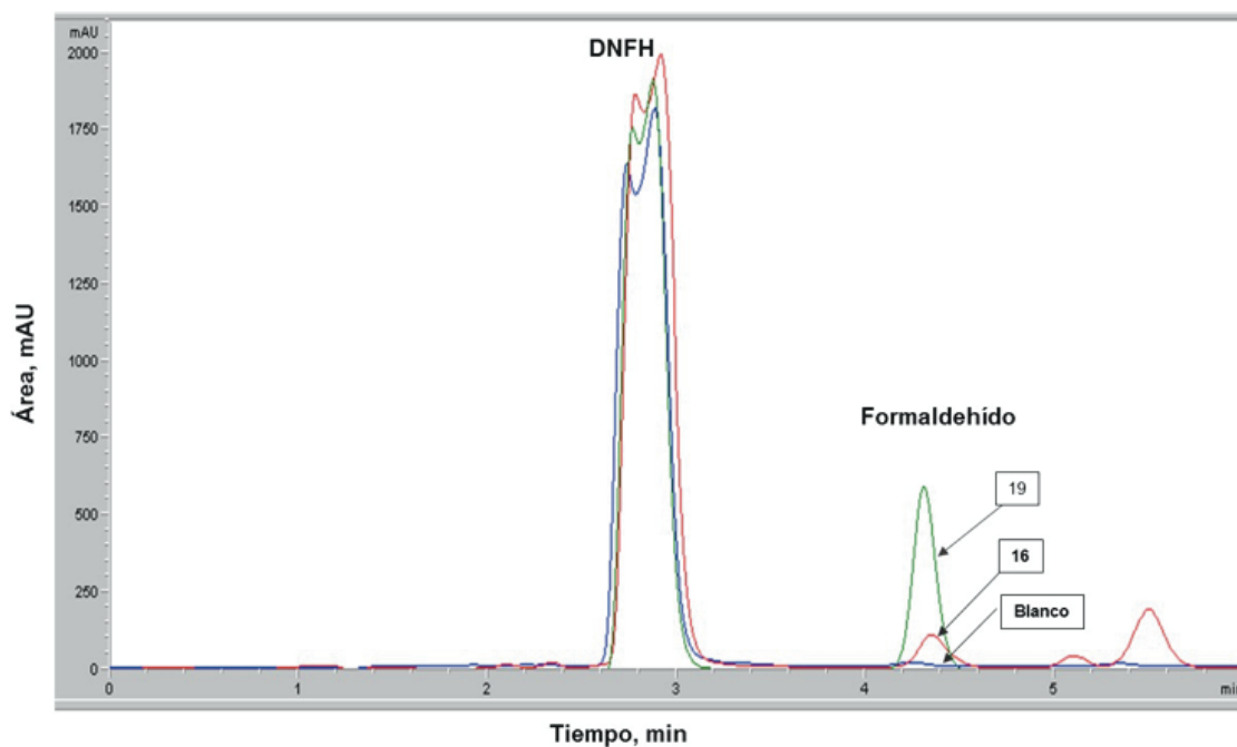
Figura 3. Ejemplo de cromatogramas obtenidos por CLAR en el análisis de formaldehído en blanco, muestra 16 y muestra 19 de los esmaltes de uñas analizadas
